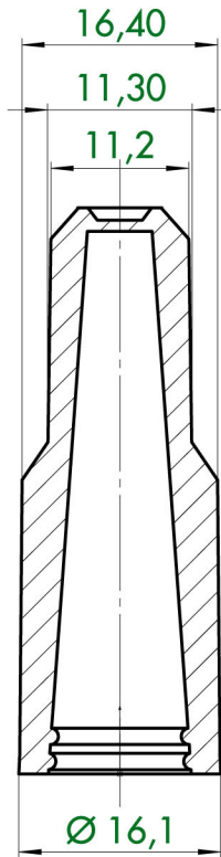
A-A
